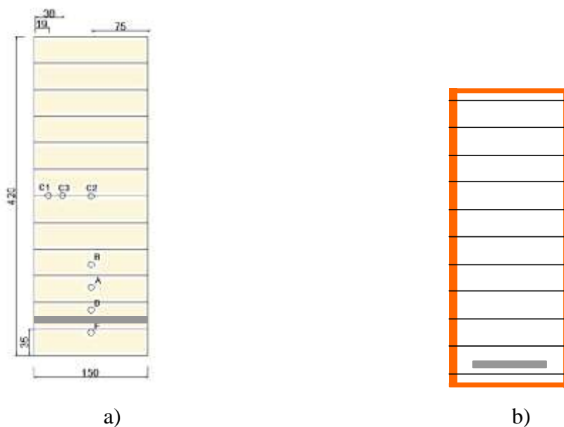
Figura 7: a) posición del refuerzo en temperatura ambiente e, b) posición posterior al fuego durante 32 minutos.
