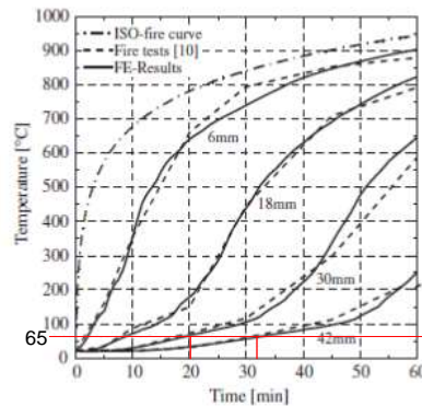
Figura 2 - Comparación de temperaturas por FE-análisis térmica e testes de fuego a diferentes profundidades de muestras de madera expuestas al fuego ISO en un lado – fuente: Frangi (2008)
